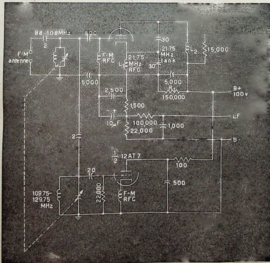
Het principe-schema der „Fremodyne“ zoals het Amerikaanse maandblad ELECTRONICS het afdruckt. Het geeft enig inzicht in hetgeen Hazeltine heeft opgezet.
